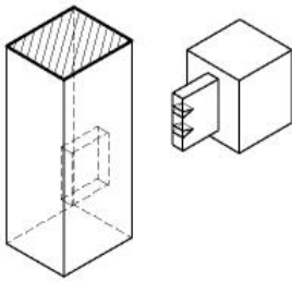
24. 지옥장부맞춤
