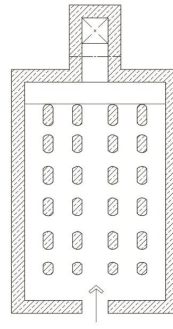
허튼고래 2
