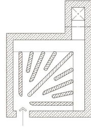
선자고래 2
