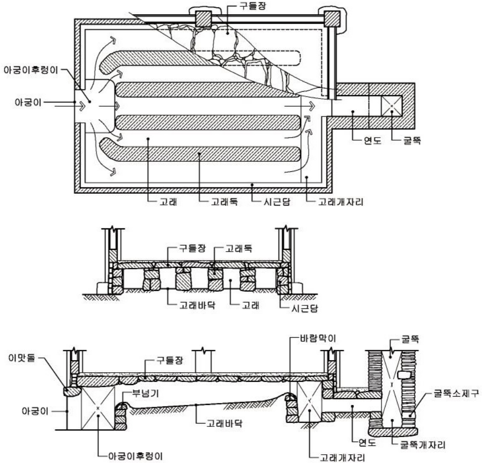
온돌의 구조(함실아궁이-민가)
