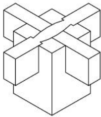
27. 내외주먹장맞춤
