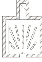
선자고래 1
