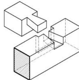
29-2. 통널고주먹장맞춤
