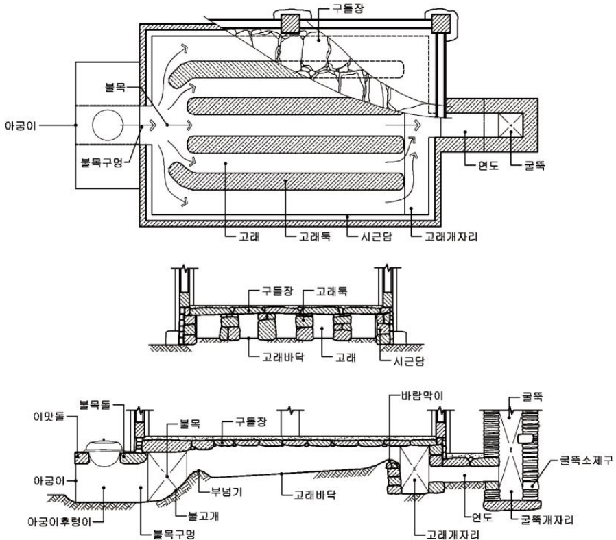
온돌의 구조(부뚜막아궁이)
