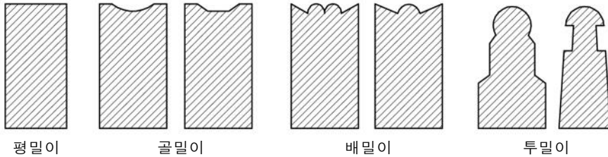
살의 모양
