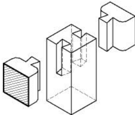
28-3. 주먹장맞춤
