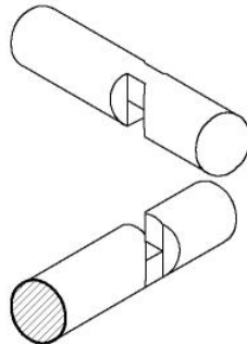
5-1. 왕지맞춤
