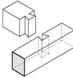
28-1. 주먹장맞춤
