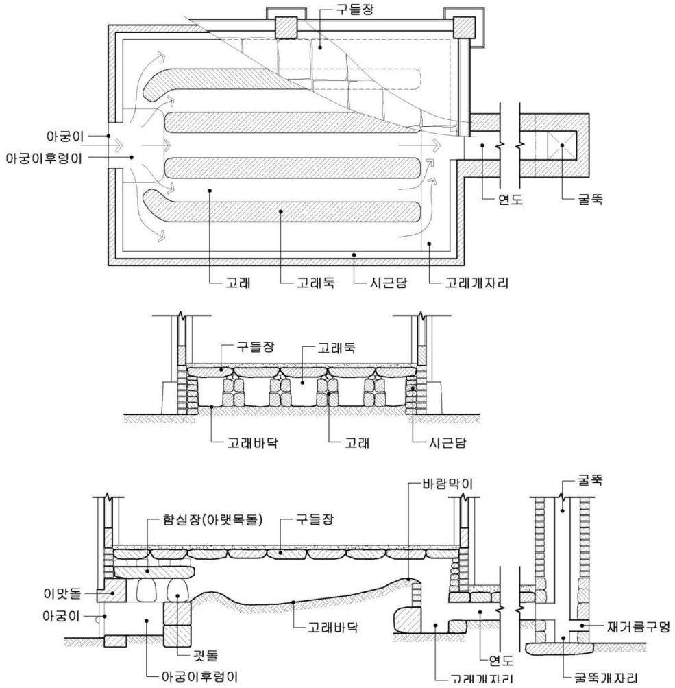
온돌의 구조(함실아궁이-궁궐)
