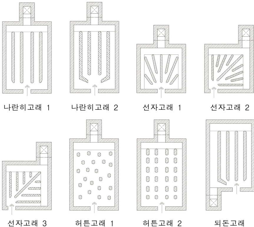
고래의 형태
