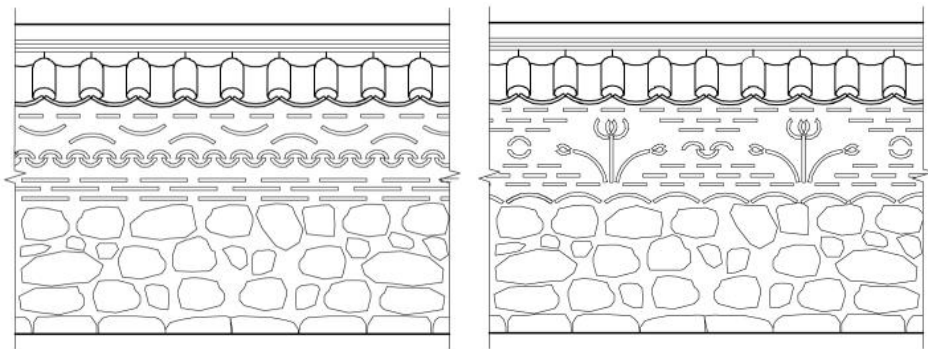
와편담(문양없음)
