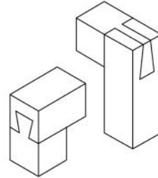
28-2. 주먹장맞춤
