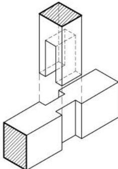
10. 가름장맞춤
