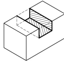
온턱파내기
