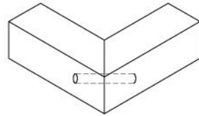
17. 연귀산지맞춤
