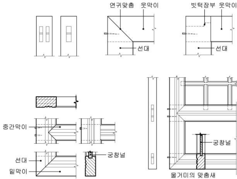
울거미의 맞춤
