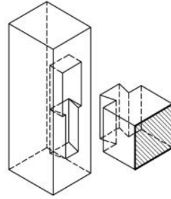
26. 내림주먹장맞춤
