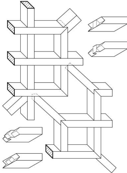
어금팔모맞춤
