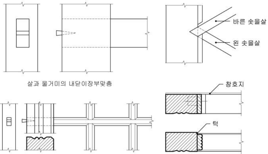
살과 울거미의 맞춤
