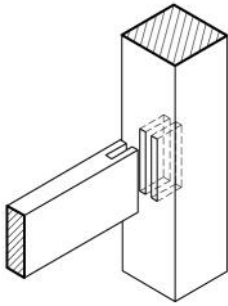
4. 쌍갈맞춤(가름장)
