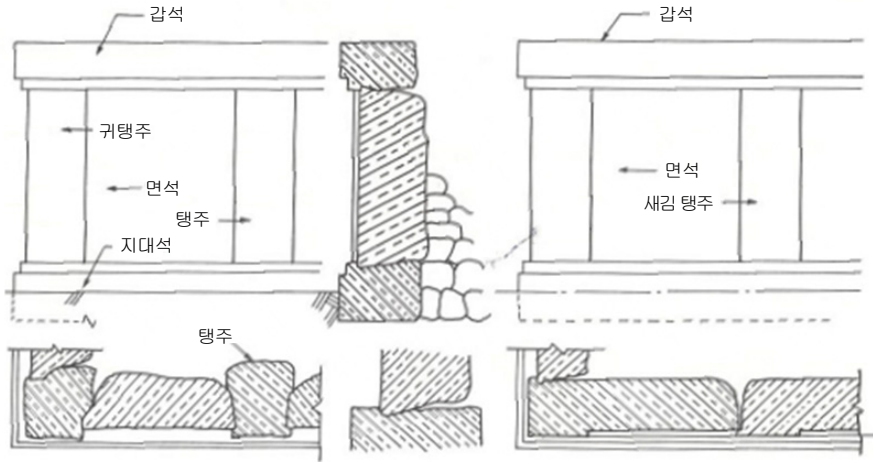
가구식기단
