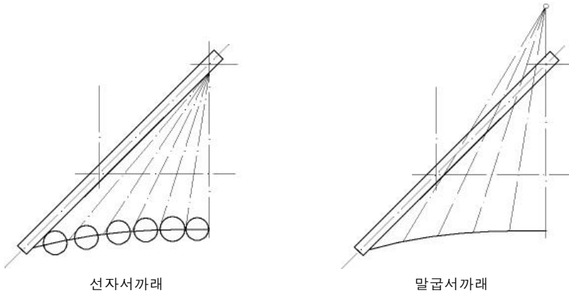
귀서까래 작도 및 배치법
