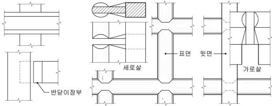
반달이장부맞춤
