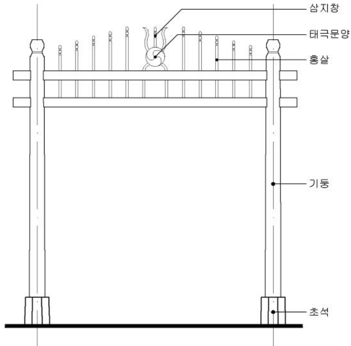
홍살문
