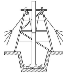
몽둥달고
