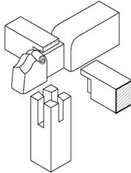
7. 화통맞춤
