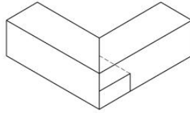
13-2. 반연귀맞춤
