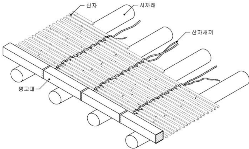
산자역기
