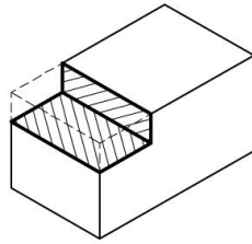
외쪽따내기
