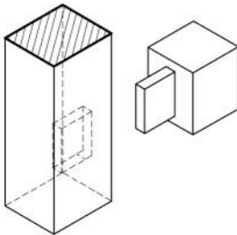
21. 세로장부맞춤
