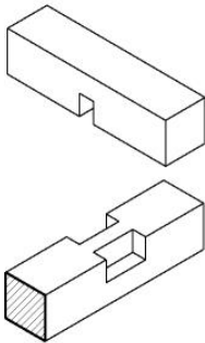
35. 양걸침턱맞춤
