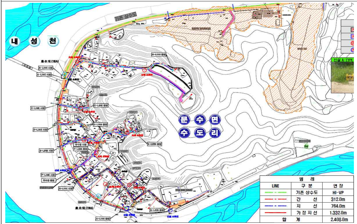
상수도관 교체 계획도
