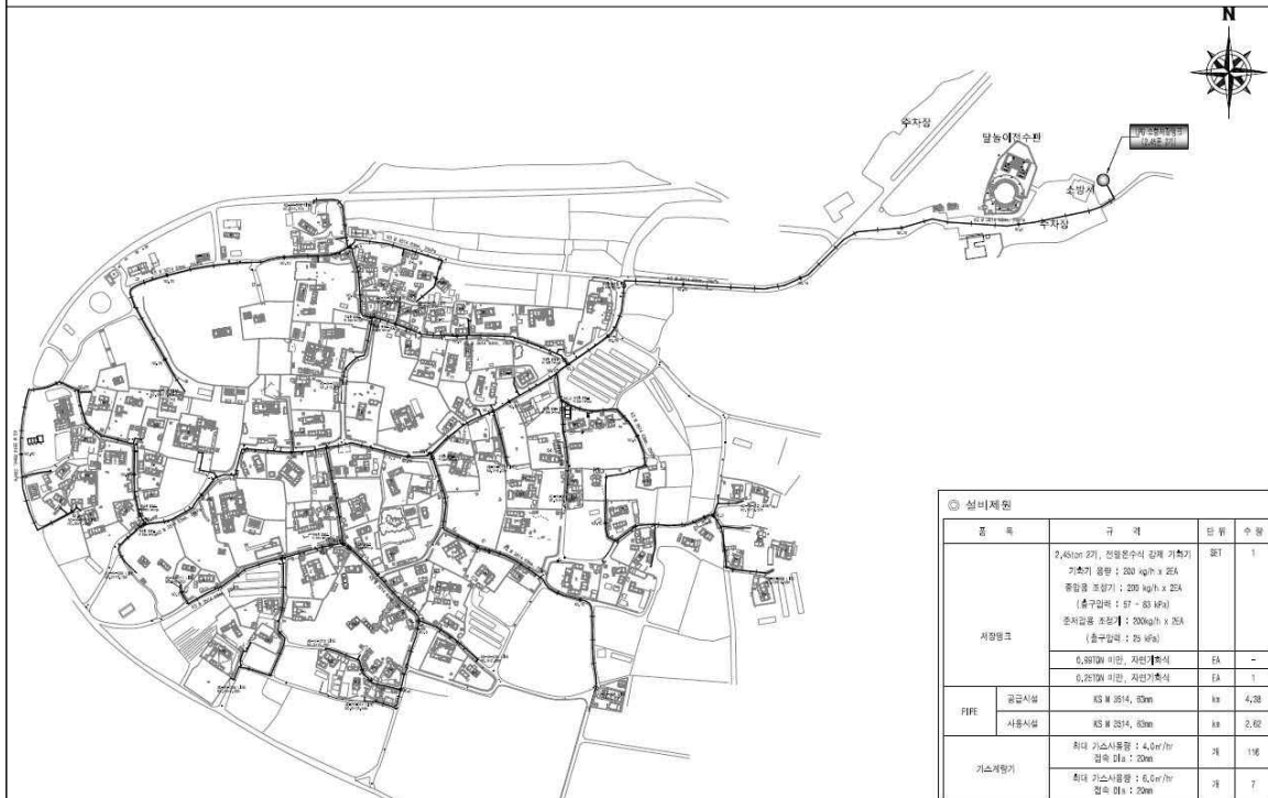
도면2. LPG배관망 구축 계획도
